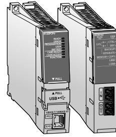
R120PCPU/R6RFM Prozess-CPU und redundantes Funktionsmodul
