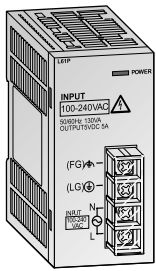
L61P Netzteil
