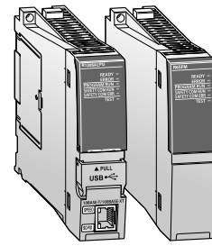
R120SF CPU/R65FM Sicherheits-CPU und Sicherheitsfunktionsmodul
